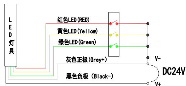
DC24V共正 (Common +)
