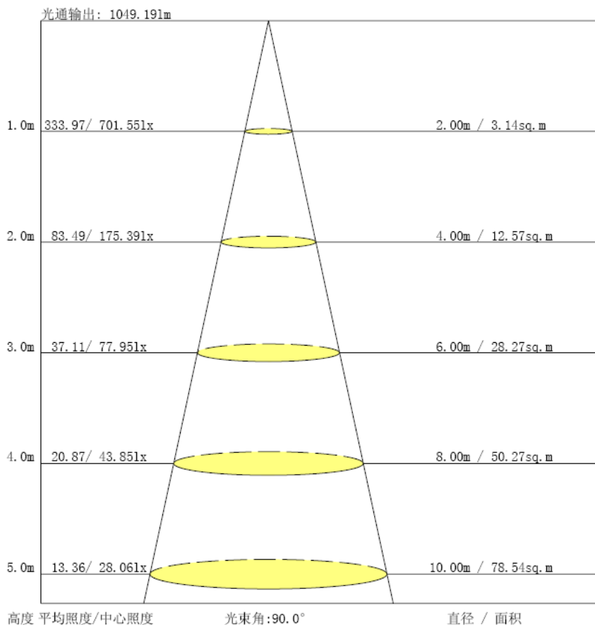
灯具有效平均照度图
