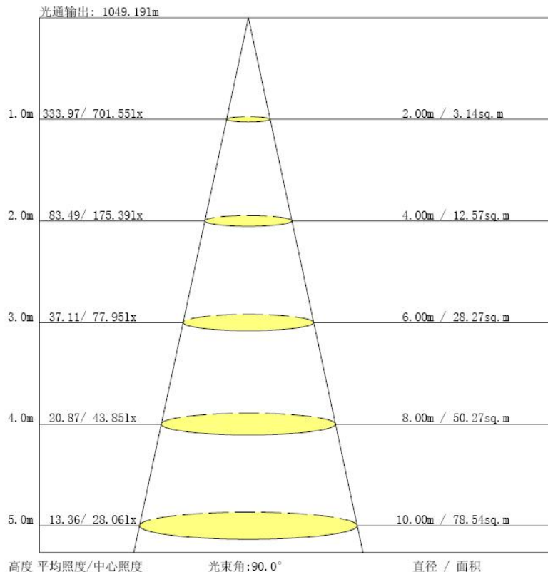
灯具有效平均照度图
