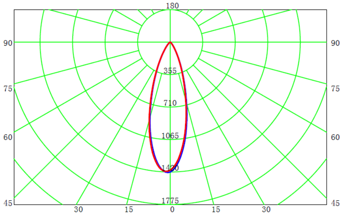
配光曲线
