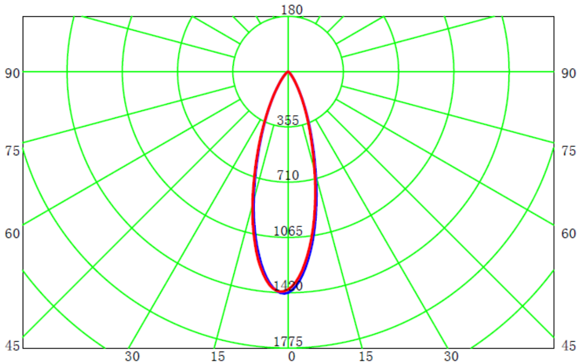
配光曲线
