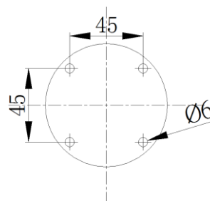
安装孔位
