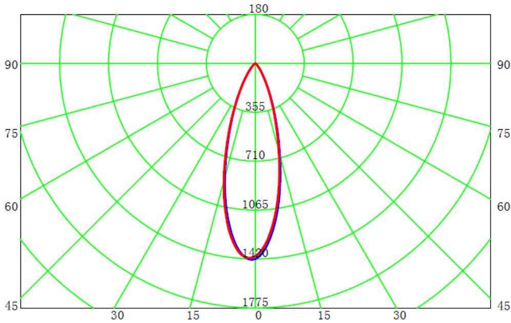
配光曲线
