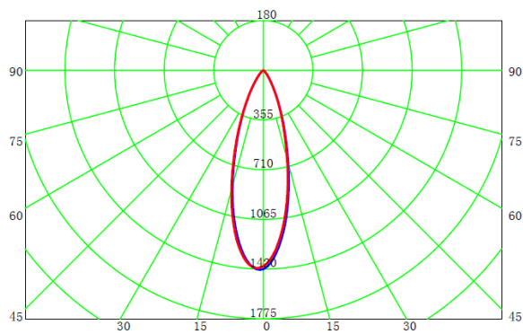
配光曲线
